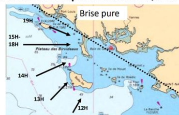
La brise thermique en baie de Quiberon
